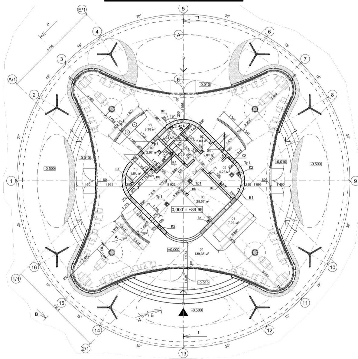
ПЛАН НА ВІДМ.0.000
